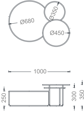
PLT10076 - PLANET ÜÇLÜ SEHPA 100x76x35h
