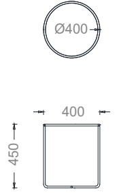
PLTQ40- PLANET YUVARLAK SEHPA ÇAP 40x45h
