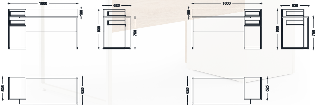
MDO60160 - MİLA- HOME OFİS MASASI SOL DOLAPLI 60x160
