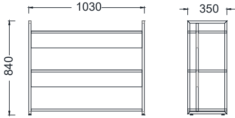
MK10384 - MİLA ÇALIŞMA KİTAPLIK 103x35x84h
