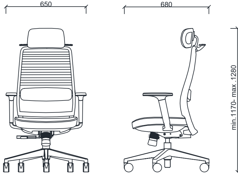
BRK54010 - LUNA YÖNETİCİ KOLTUĞU
