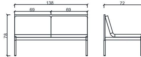
BRK3055-Unit İkilii Orta
