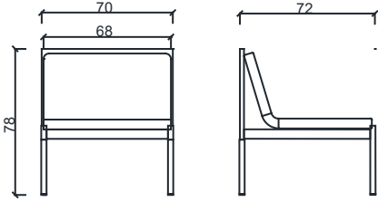
BRK3050-Unit Tekli Orta
