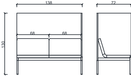
BRK3154-Unit İkilı Sağ Köşe
