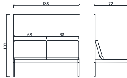
BRK3155-Unit İkilı Orta
