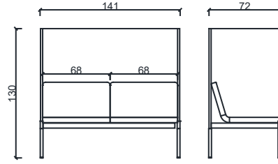
BRK3152- Unit İkilı
