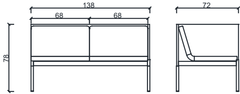
BRK3054-Unit İkilii Sağ Köşe
