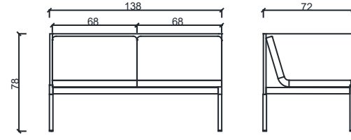
BRK3053-Unit İkilii Sol Köşe
