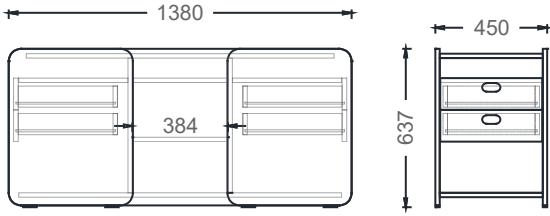
M2C14045 -MİO İKİ ÇEKMECELİ ÇALIŞMA GRUBU ETAJER 140cm
