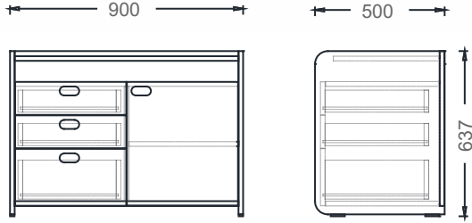
MCA9050 - MİO ÇEKMECELİ SAĞ YAN DOLAP
