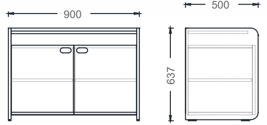
MK9050 - MİO KAPAKLI YAN DOLAP
