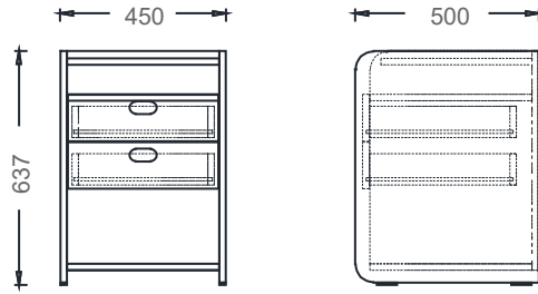
M2C4550 - MİO İKİ ÇEKMECELİ KESON
