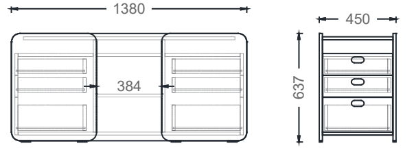
M3C14045 -MİO İKİ ÇEKMECELİ ÇALIŞMA GRUBU ETAJER 140cm
