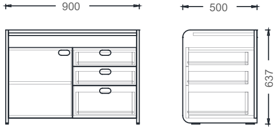
MCO9050 - MİO ÇEKMECELİ SOL YAN DOLAP
