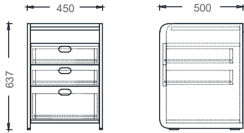
M3C4550 - MİO ÜÇ ÇEKMECELİ KESON
