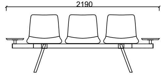
BRK2243S2 - BEST ÜÇLÜ BEKLEME İKİ YAN SEHPALI
