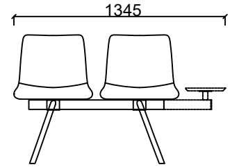
BRK2242S1 - BEST İKİLİ BEKLEME TEK YAN SEHPALI
