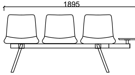
BRK2243S1 - BEST ÜÇLÜ BEKLEME TEK YAN SEHPALI
