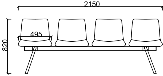
BRK2244 - BEST DÖRTLÜ BEKLEME
