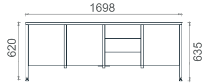
MLA50170 Mila Sađ Uzun Etajer 170x50x64h
